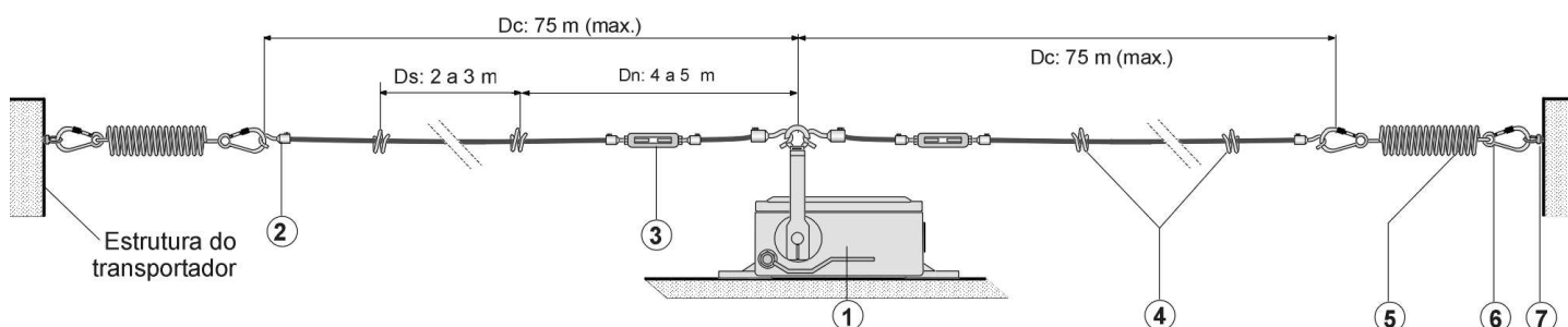
Fig. 1 – diagrama de montagem da chave com os acessórios
