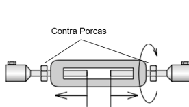
Fig. 2 – abrir esticador
