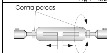
Fig 2 - Abrir esticador
