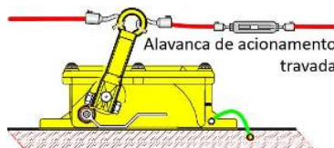
Fig. 9 - Chave travada na emergência
