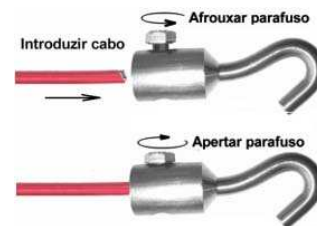
Fig. 6 - fixação do cabo no gancho
