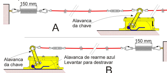
Fig. 7 - ajuste da mola tracionadora
