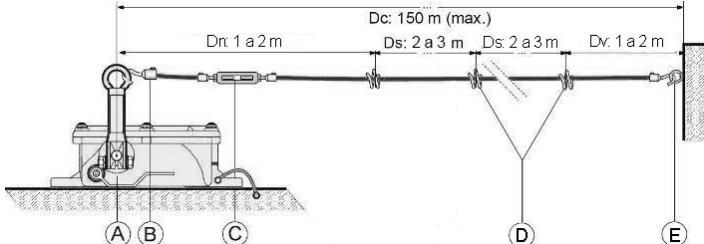
Fig. 3 – Montagem com componentes de montagem rápida
