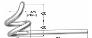
Fig. 1 – Suporte para cabo de aço
