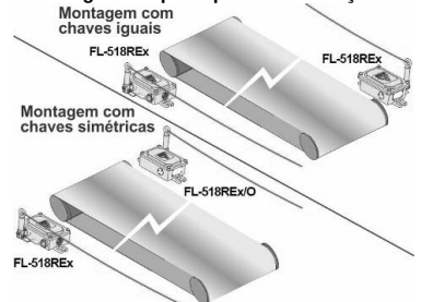
Fig. 2 – Montagem das chaves iguais ou simétricas
