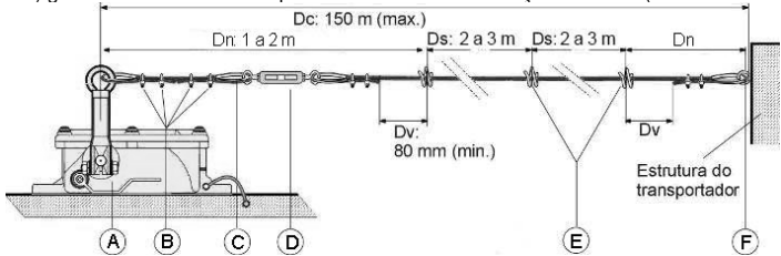
Fig. 4 – Montagem com componentes convencionais
