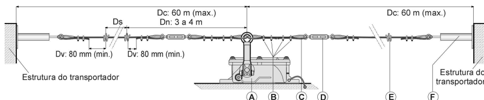
Fig. 3 - Instalação com componentes convencionais e tracionadores
