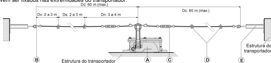
Fig. 2 - Instalação com componentes de montagem rápida
