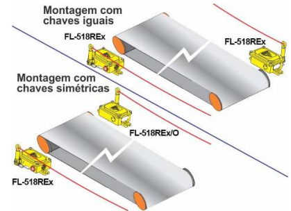
Fig. 2 - Montagem das chaves iguais ou simétricas
