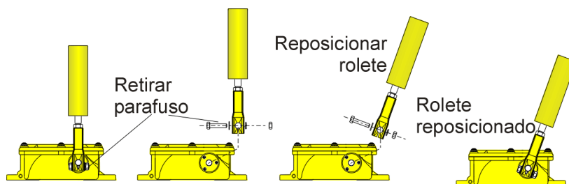
Fig.4 reposicionamento do rolete
